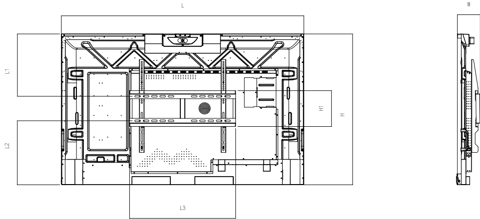
比例 1:10
